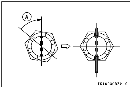
A. 時計回りに回す
